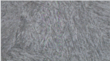
太阳耐磨件斗齿的微观结构
